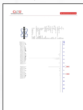
QNMR
